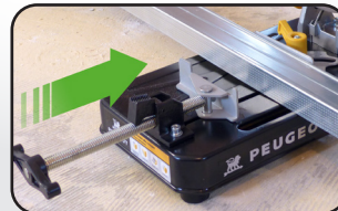
Presse à réglage rapide Quick clamp
